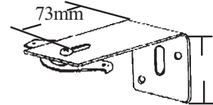
Face Fix Wall Bracket (Proj 70mm) 8055
